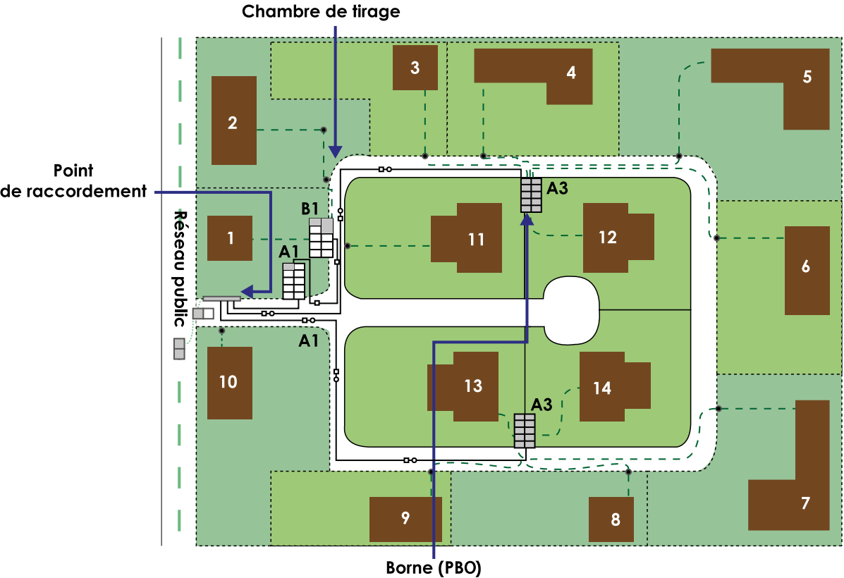
Fig 92 : Diagramme de câblage pour un lotissement
