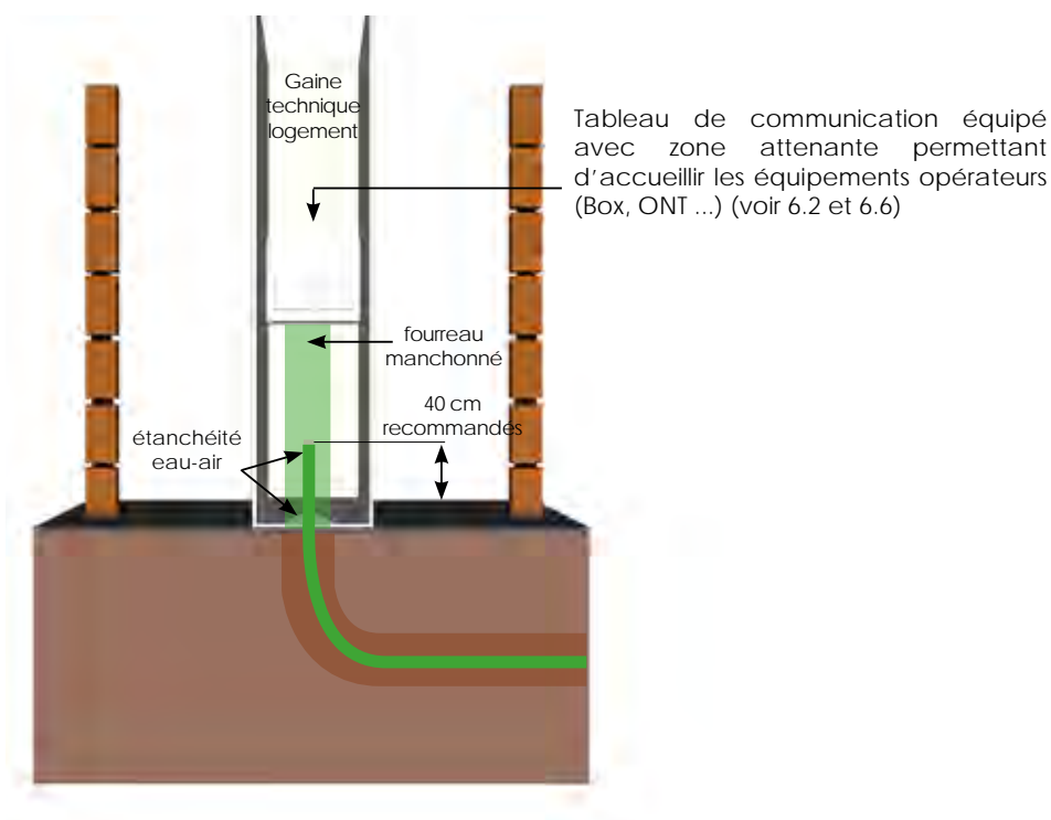
Fig 25 : Cas particulier des locaux individuels (logements ou locaux à usage professionnels)
