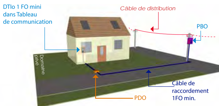
Fig 33 : Local individuel isolé* sur terrain, avec raccordement souterrain à un PBO
